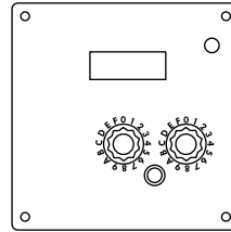
11 – ASCII Seite 30
