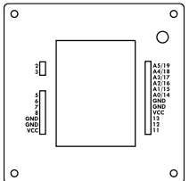
99 - Prototyp Seite 41
